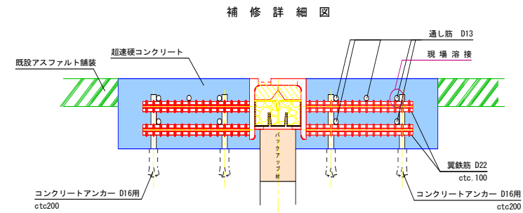
伸縮継手装置設置工（プロフジョイントSW-60）
