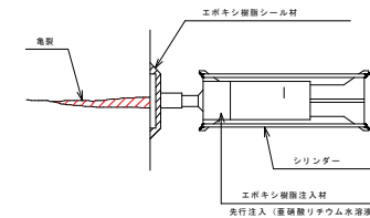
ひび割れ補修工 (主桁・橋台) 詳細図
