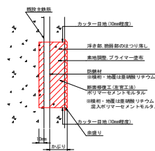
断面修復工 左官工法 (主桁・横桁・地覆・橋台) 詳細図
