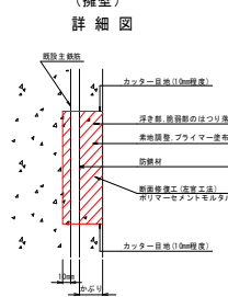
断面修復工 左官工法 (換壁) 詳細図
