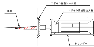
ひび割れ注入工 (主桁・地覆・橋台) 詳細図
