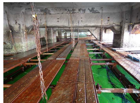
足場工完了 ↓
